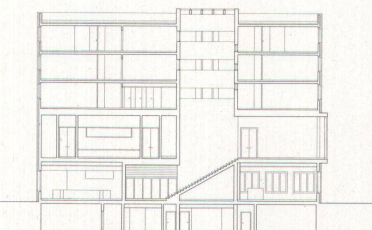
Der Querschnitt zeigt die Beziehung von der Eingangshalle zum Foyer und dem Lichthof
