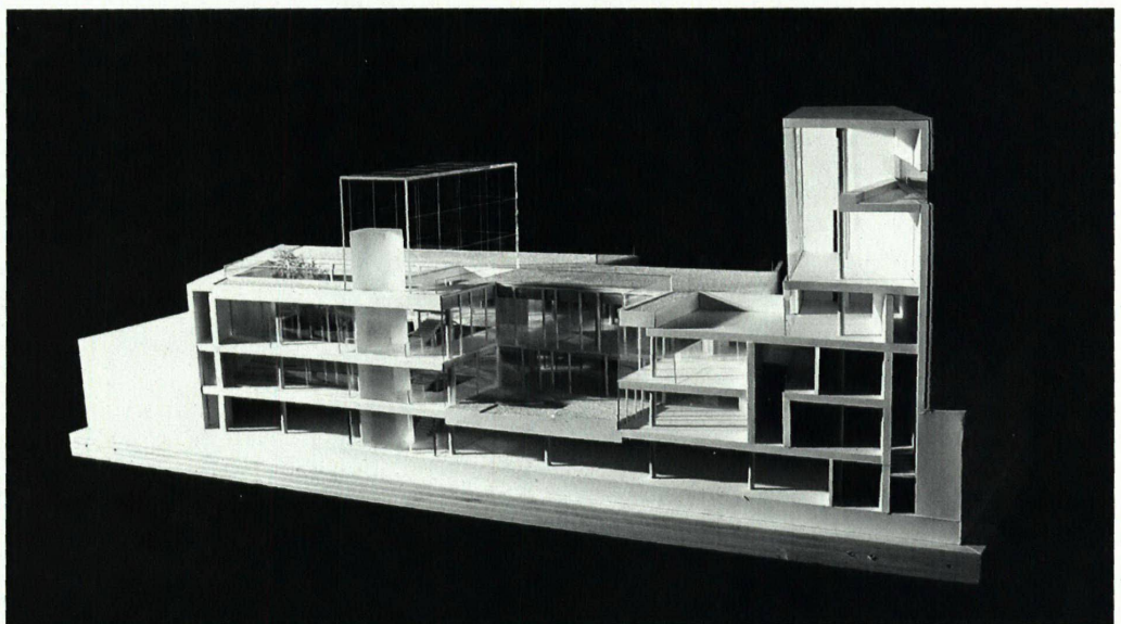
Längsschnitt. Die Platte steigt von zwei auf drei Geschosse an, das Gelände sinkt um ein halbes, das architektonische U-Boot taucht aus dem Boden auf
