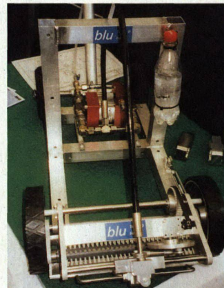
Die Schneideinheit des Wasserstrahlmähers. Zum Design der Verschaltung hats nicht mehr gereicht
