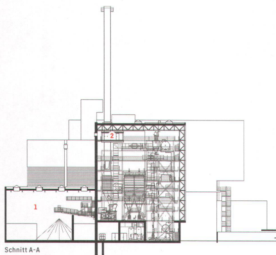
Schnitt A-A
