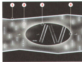
1-2 Querschnitt und Deckenplan. Lichtband 1 , Grundbeleuchtung 2 , LED-Beleuchtung 3 , Hinterleuchtung 4 . Pläne: Reflexion
