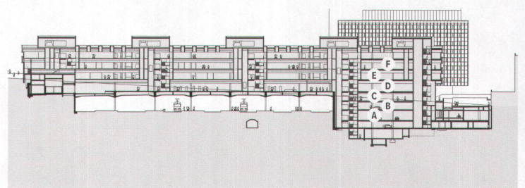
Schnitt A-A
