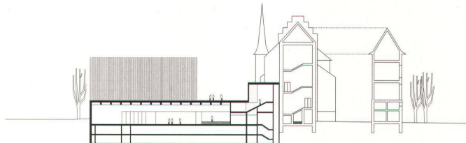
^ Längsschnitt: Unter der Halle liegen die Kulturgüterschutzräume.
