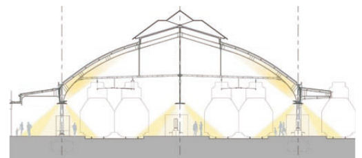
^ Der Querschnitt zeigt die Wirkung der Leuchten und den präzisen Lichtverlauf.
