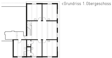
<Grundriss 1. Obergeschoss
