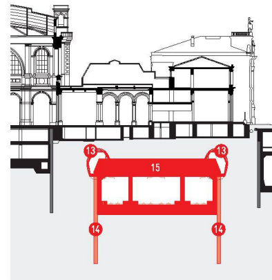
^Querschnitt durch das alte Bahnhofgebäude und den neuen Tiefbahnhof.
