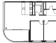
<2_Standardwohnung 3 ½ Zimmer neu: 90 m².
