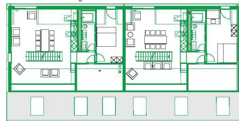
Grundriss 2. Dachgeschoss.
