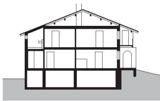
Querschnitt | Section
