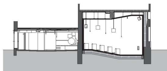
Längsschnitt | Longitudinal section
