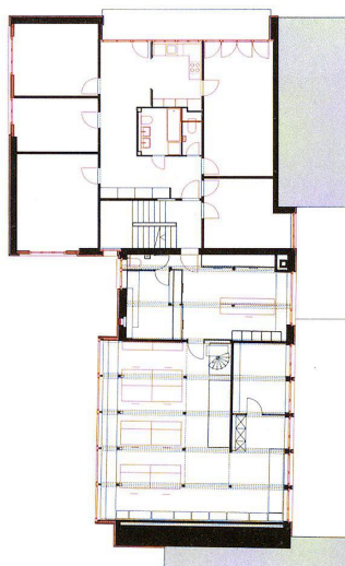
2. Obergeschoss des Wohnhauses, Hauptgeschoss des Ateliers.
