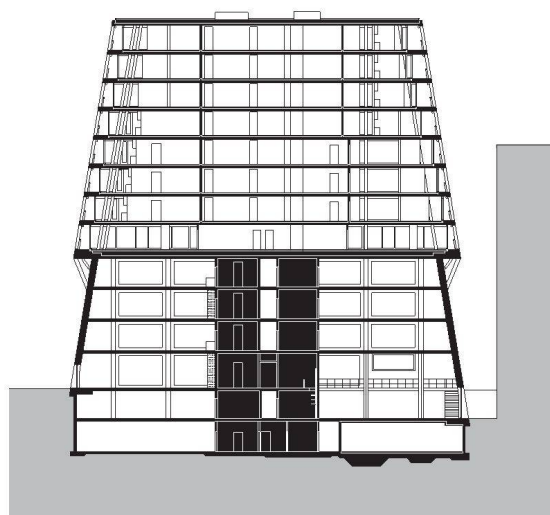
Längsschnitt
