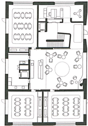
Erdgeschoss
