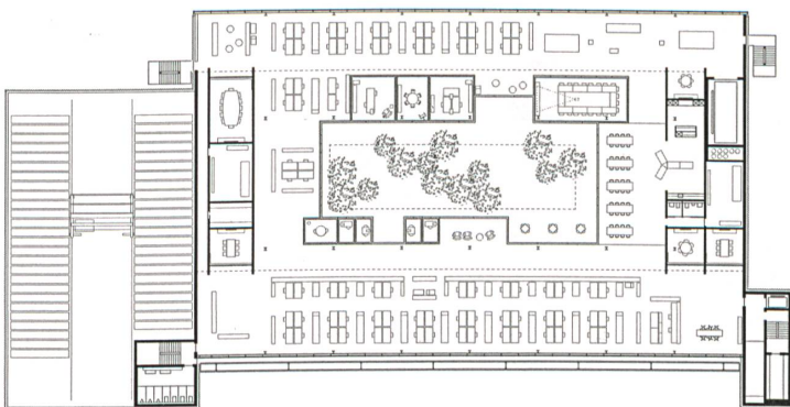
Grundriss Bürogeschoss.
