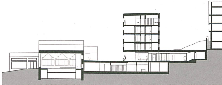
Querschnitt
