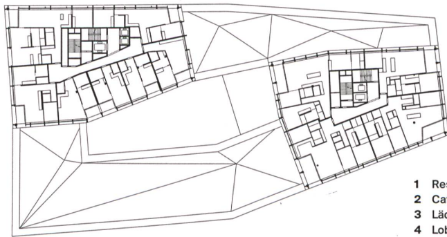
8.-11. Obergeschoss
