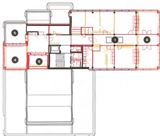
4. Obergeschoss
