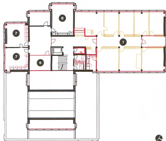
2. Obergeschoss
