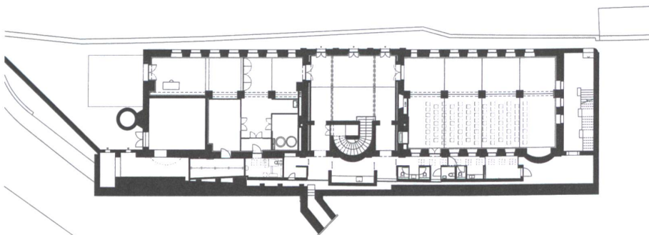
Untergeschoss: der Theatersaal rechts, der Hautechnik- und Servicegang vorne.
