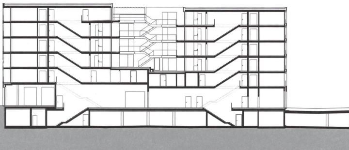
Längsschnitt
