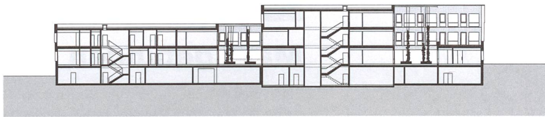
Längsschnitt
