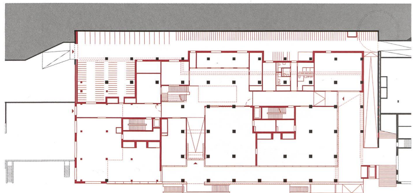
Oberes Hofgeschoss
