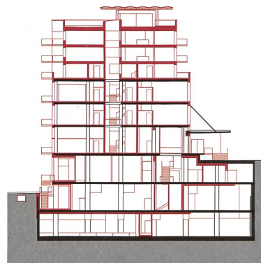
Querschnitt
