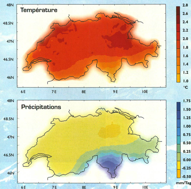
Scénarios climatiques pour l'hiver: modifications possibles autour de l'année 2050 par rapport au climat de la période 1931-1980.
