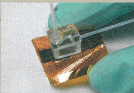
Prototype d'un transistor organique capable de résister à des environnements naturels corrosifs.
