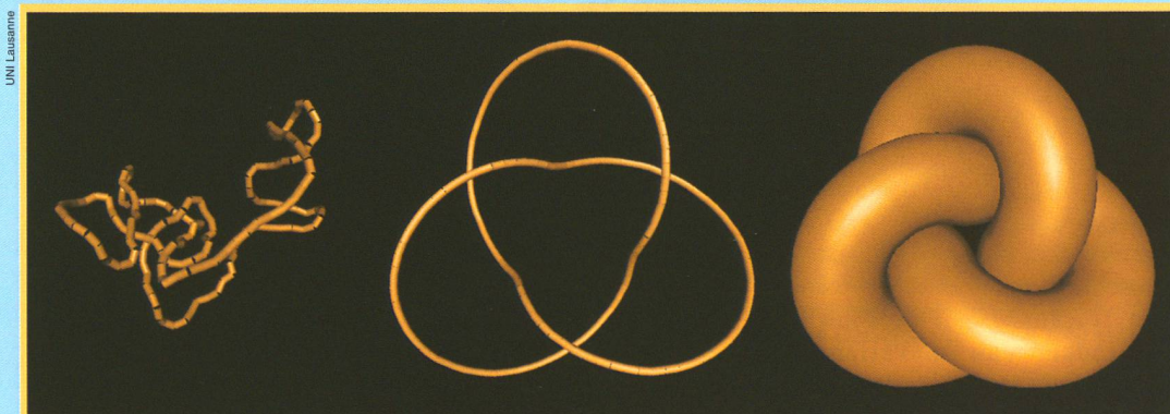
Der verschlungene DNS-Strang einer Bakterie. Um welchen mathematischen Knoten könnte es sich handeln?
