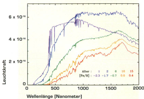
Galaxie-Spektrum: Die Kurven zeigen, wie Sterne entstehen und vergehen, und sich damit die chemische Zusammensetzung der Galaxie ändert.
