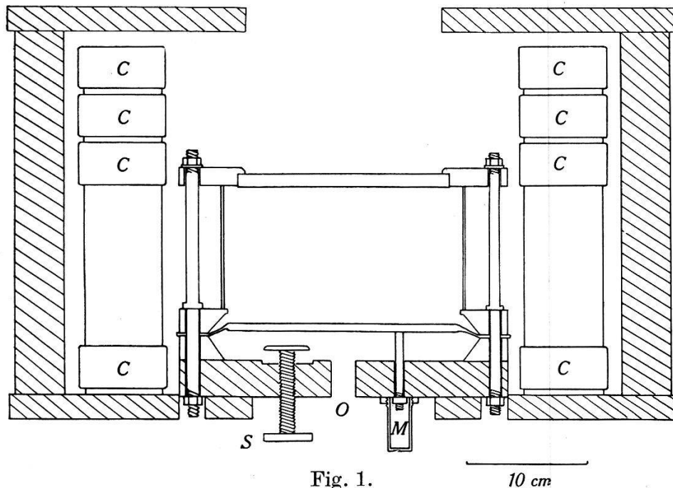
Fig. 1. Schnitt durch die Wilsonkammer, Feldspulen C und Eisenarmatur (schraffiert). Von den acht Säulen, die die Deckplatte tragen, sind im Schnitt nur zwei gezeichnet.
