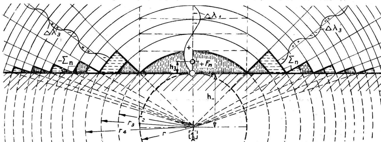
Fig. 2. Plan critique, segment d'anneau-quart-d'onde, antennes spatiales.
