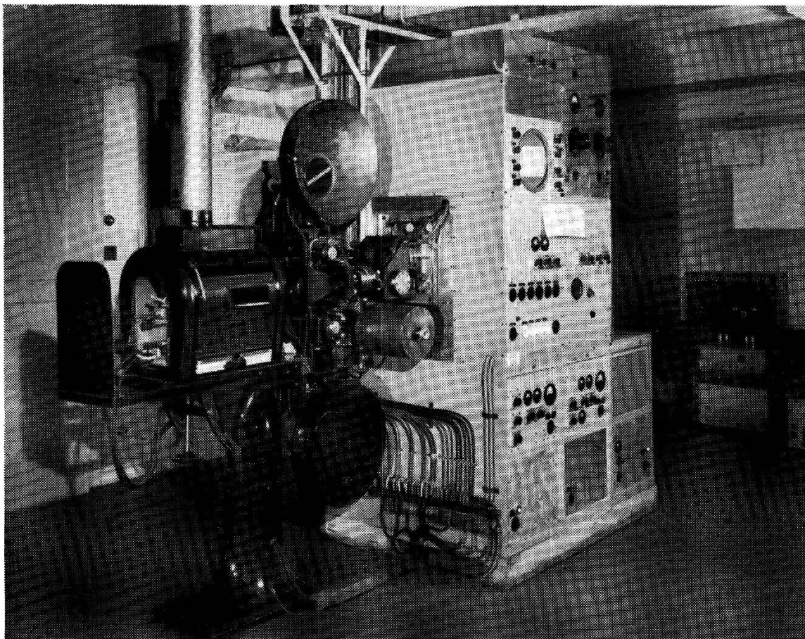
Fig. 3. Filmabtaster.
