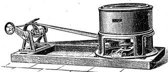
Centrifugal-Trockenmaschine.
