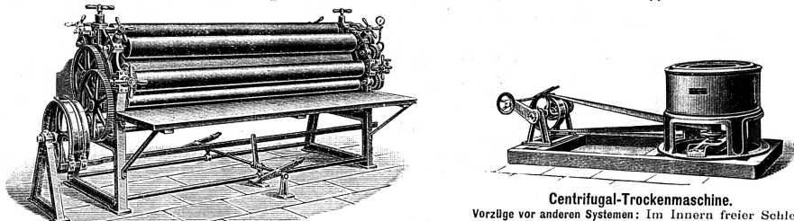
Dampfmangel-Trocken- und Plättmaschine für glatte Wäsche in 4 verschiedenen Längen, mit Heizcylinder von 500 mm Durchmesser, 4 Andruck- u. 1 Ablegewalze, mit höchster Leistung u. Vollkommenheit.
