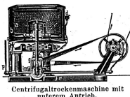
Centrifugaltrockenmaschine mit unterem Antrieb.
