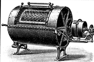
Doppeltrommel-Waschmaschine.
