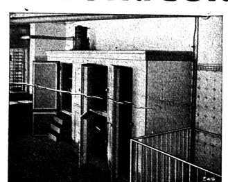
Autofrigorkühlanlage im Hotel Schweizerhof Luzern.
