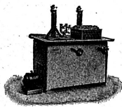
Universalmaschine „SIMPLON“ Grösse 1
