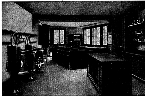
Elektrische Küche Hotel Urnerhof & Stern, Fläelen, für 500 Personen Leistung (2 Herde, 2 Kippessel, 2 Pâtisserie-Öfen, Bratpfanne und Wärmeschrank = 137 kW, Boiler und Durchlaufrührer für Küche, Bad und Toiletten = 27,5 kW, installiert im Jahre 1931).
