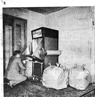
1 Flaschenzertrümmerer der Fa. Kisag AG, Bellach. Durch die Einfüllöffnung wird die Flasche in den Apparat geworfen, der dann in Gang gesetzt wird. Und im darunterstehenden Sack wird der Flaschengrüss für den Abfalltransport gesammelt.
