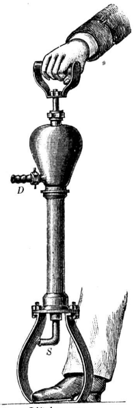
Filtrirpumpe. (1/6 natürliche Größe.)
