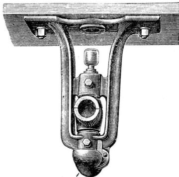
Geschlossenes Hänglager
