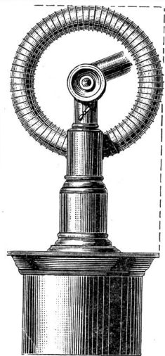
Ofensäule mit messing. Kapitalen, Kreisrohr, Messingkapsel und Ofenklappe. Wird auch bloß mit einem Ofensäulen-Aufsatz geliefert; zweckmässig für niedere Zimmer.
