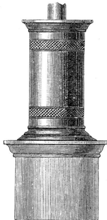
Ofensäule mit Doppel- mantel, Luftzirkulation und drei Rauchzügen.
