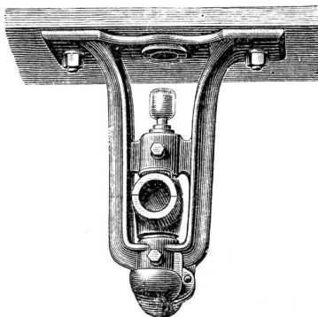
Geschlossenes Hängelager
