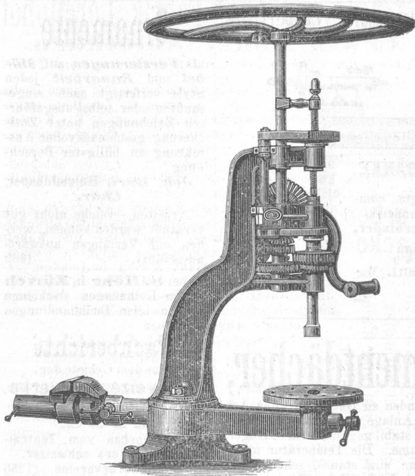
Tischhänder-Bohrmaschine für Hand- und Kraftbetrieb mit drehbarem, horizontal verschiebbarem Tisch und Parallelschraubstock, zweifacher Ueberführung, zwei Geschwindigkeiten und Selbstschaltung.
