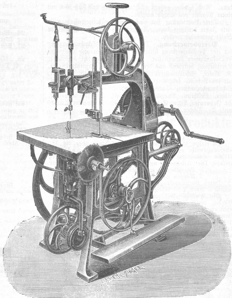
Universal-Holzbearbeitungs-Maschine.
