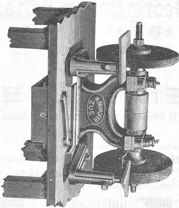
Schmirgel-Schleifmaschine mit niederem Eisengestell für zwei Schmirgel-scheiben, zwei verstellbaren Auflagen u. ohne Holzgestell. Für Schleifereien, Schlosser und Schmiede.
