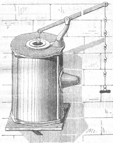
Eineylindriges doppelblasendes Gebläse zum ziehen für Schmiede, Schlosser, Chemiker etc. In 3 Grössen.
