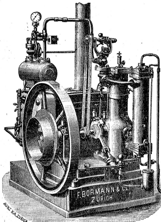
Der Motor liefert als Nebenprodukte kostenfrei: Warmes sauberes Wasser und Abdampf f. Heizungswecke.
